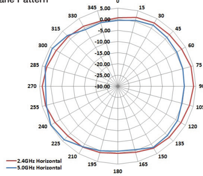
H-Plane Pattern
