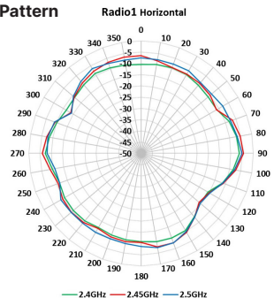
H-Plane Pattern
