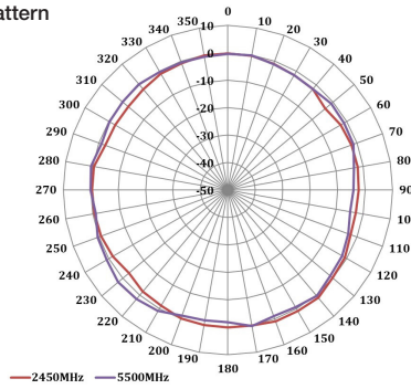
H-Plane Pattern
