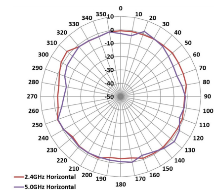
H-Plane Pattern
