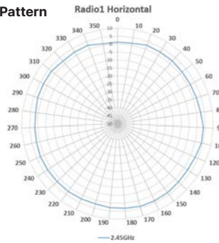
H-Plane Pattern
