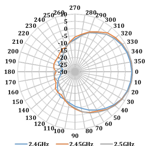
Radio1 - Vertical
