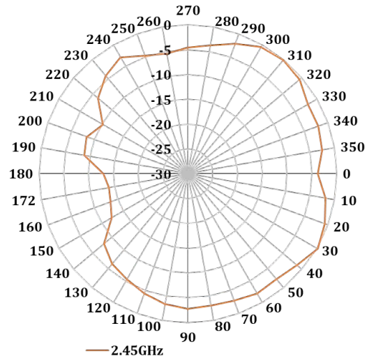
BLE antenna - Vertical
