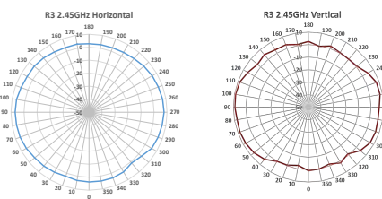
FAP-433G Radio3 antenna plots
