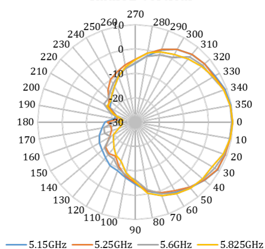
Radio2 Vertical
