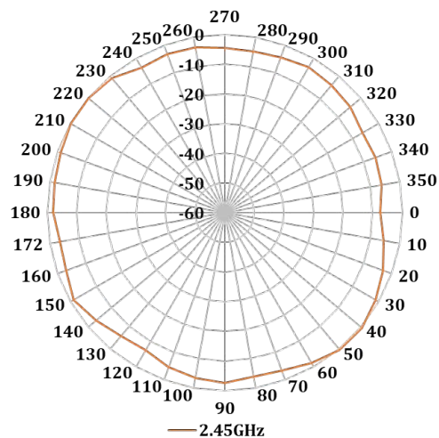
BLE antenna - Horizontal
