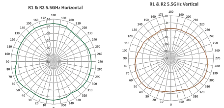
Radio3 2.4GHz plots
