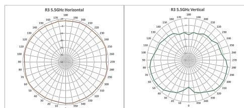
FAP-433G Radio3 antenna plots
